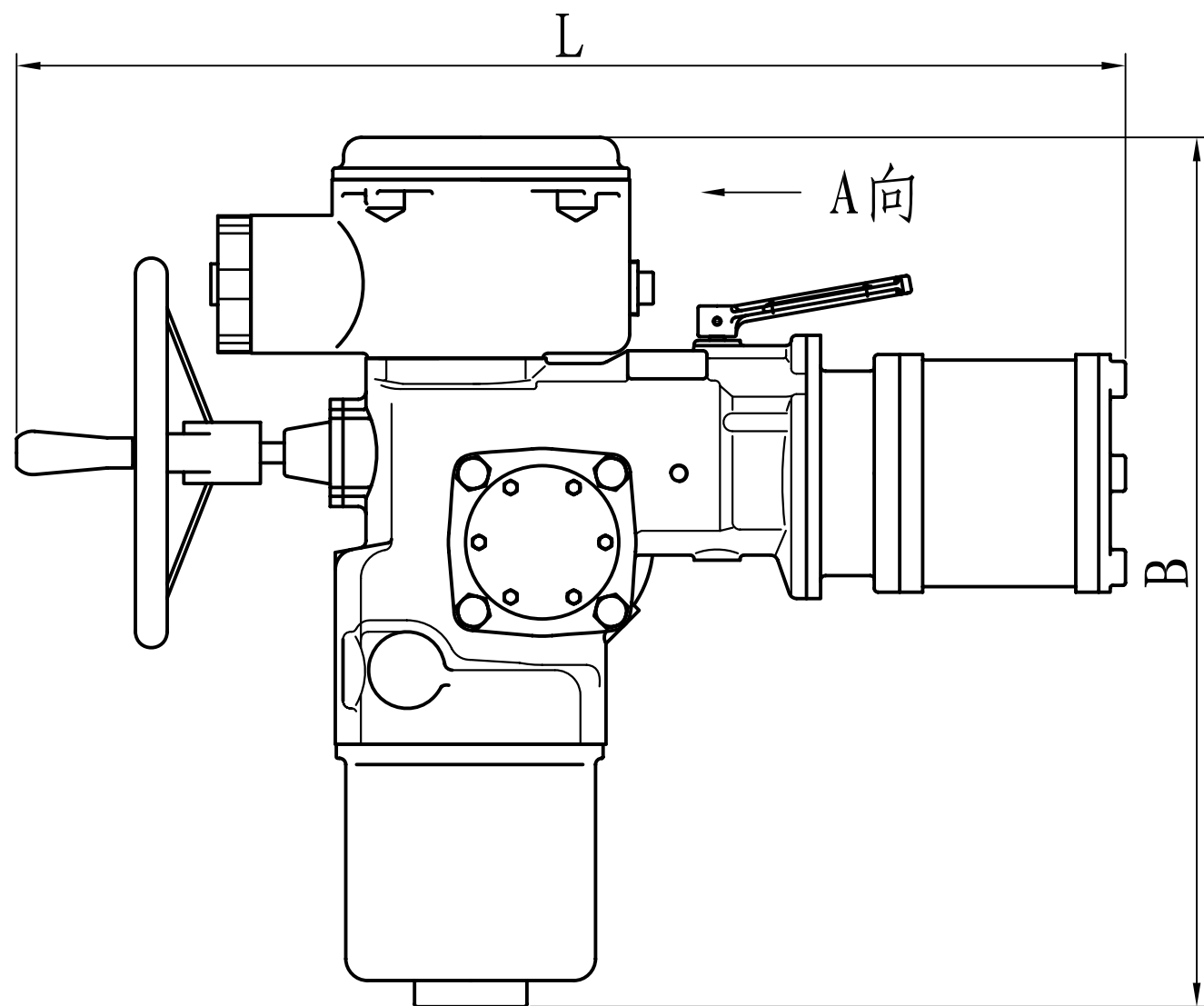
SMC-00 ~ 2. D 普通带灯盒外形尺寸
